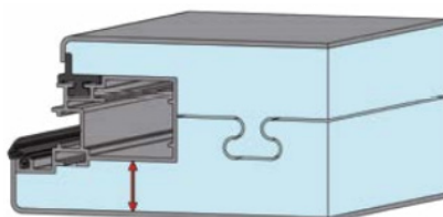
Coupe de l'ouvrant SOLOBLOC 80.2 bénéficiant du brevet \Omega méga d'ISOSTA
