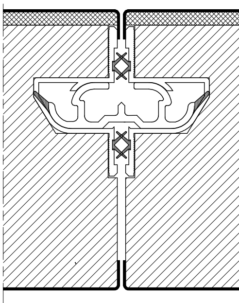
EPAISSEUR 85 mm AST PREMIUM
