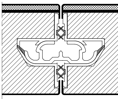
EPAISSEUR 55 mm AST CONFORT
