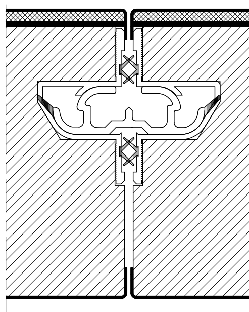
EPAISSEUR 85 mm AST CONFORT
