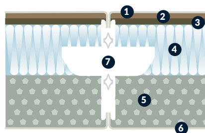
ELS ULTRA autoportant
